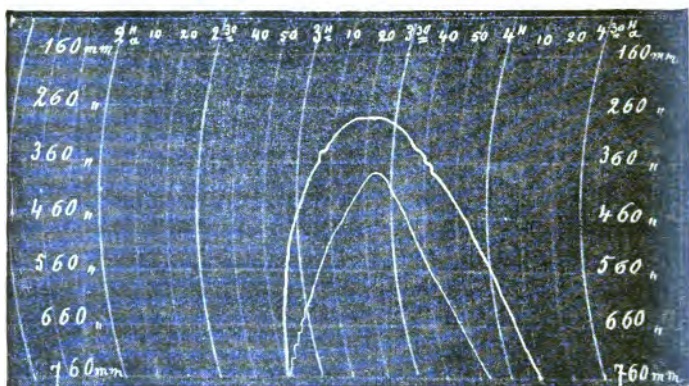
Courbes barométriques des ballons-sondes allemands dans l'expérience du 14 novembre 1896. La grande courbe est celle du Strassburg et la petite celle du Cirrus de Berlin.
